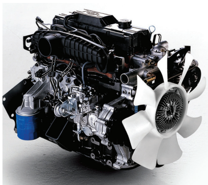
Motor 2.5 L Turbodiesel Intercooler 16 Válvulas. Potência máxima: 130,5 cv / 3.800 rpm - Torque máximo: 26 Kgm / 1.500 rpm
